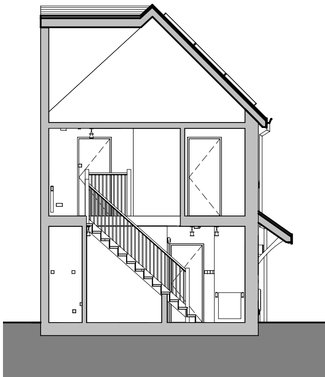
SECTION 1 : 100
