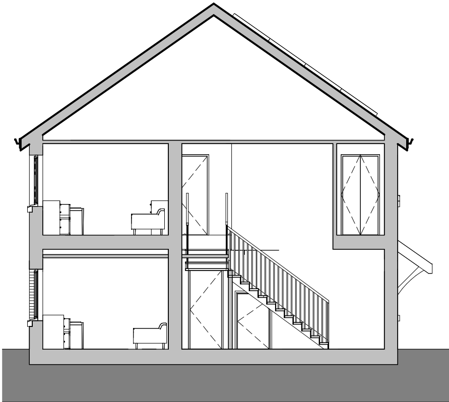
SECTION 1 : 100
