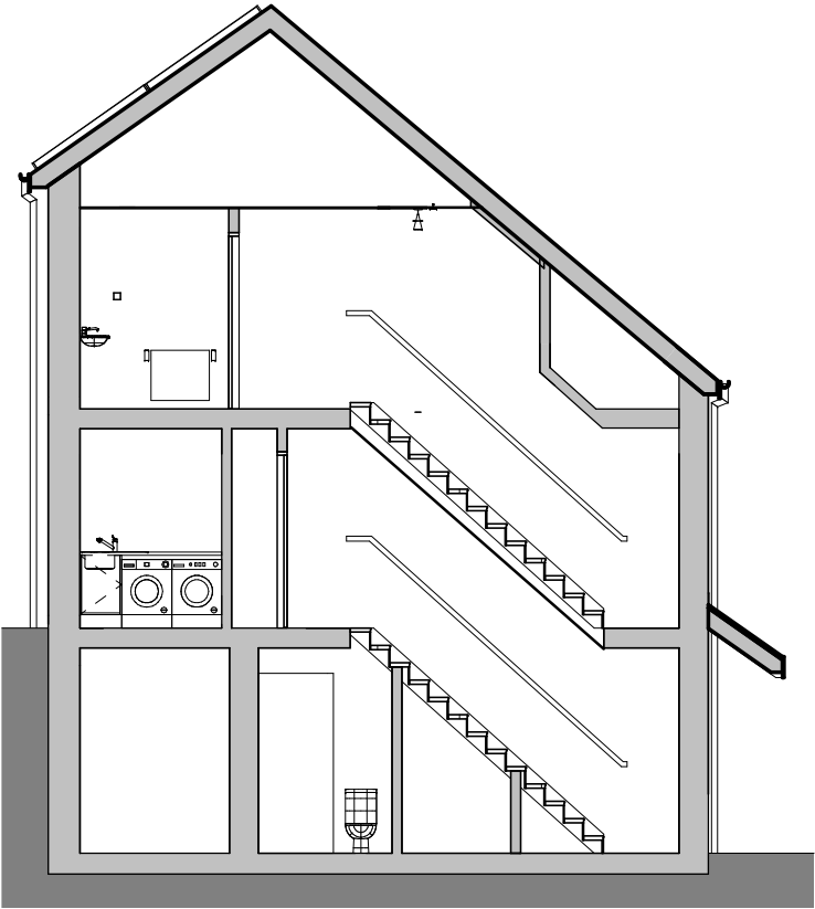
SECTION 1 : 100
